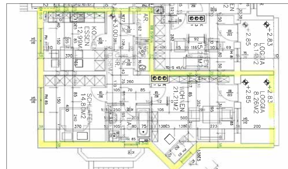
Plan Wohnung Nr II/1/6
