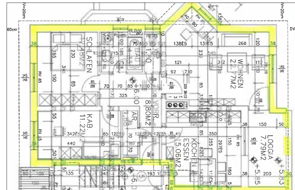
Plan Wohnung Nr I/2/5
